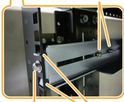
机柜后侧固定螺钉 (同捆M5 螺钉、 一个滑动角架单元 配两枚螺钉)
