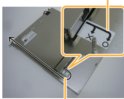
螺栓
