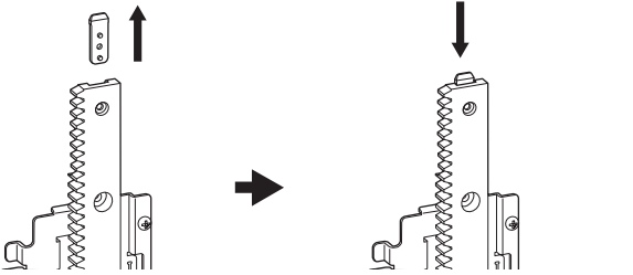
安装在最上层单元
