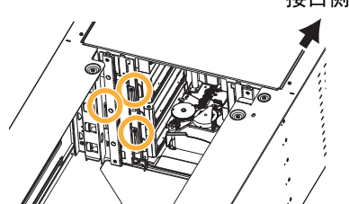
接口侧左升降导轨
