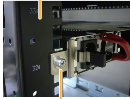
机柜前侧固定螺钉 (同捆M5 螺钉、一个滑动 角架单元配两枚螺钉)
