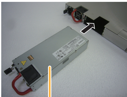
电源单元
