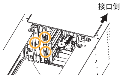
接口侧左升降导轨
