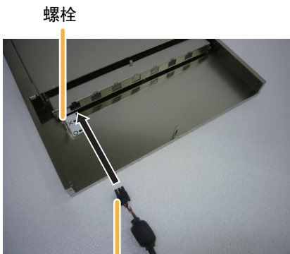
DC 电源线的插头
