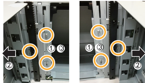
接口侧的左侧升降导轨
