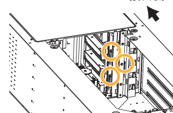
接口侧右升降导轨
