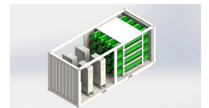
集装箱式氢能燃料电池系统
